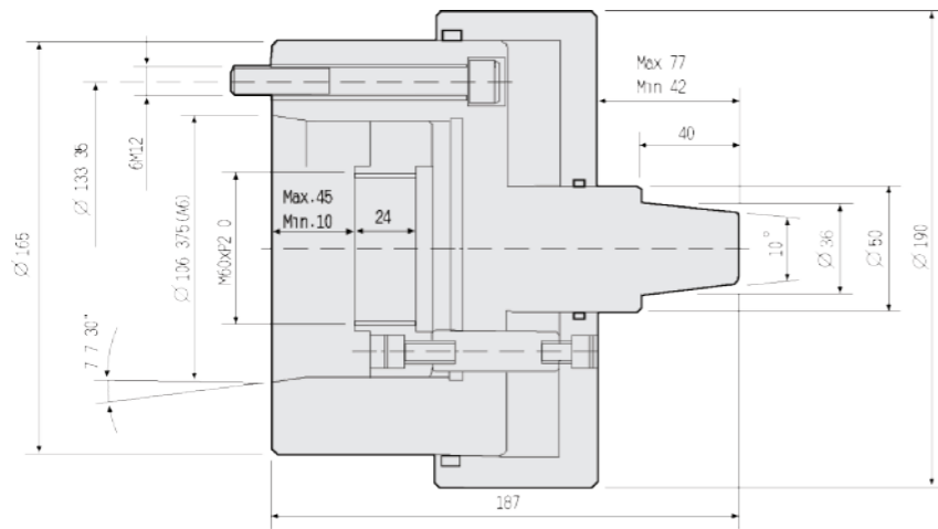
產品示意圖
